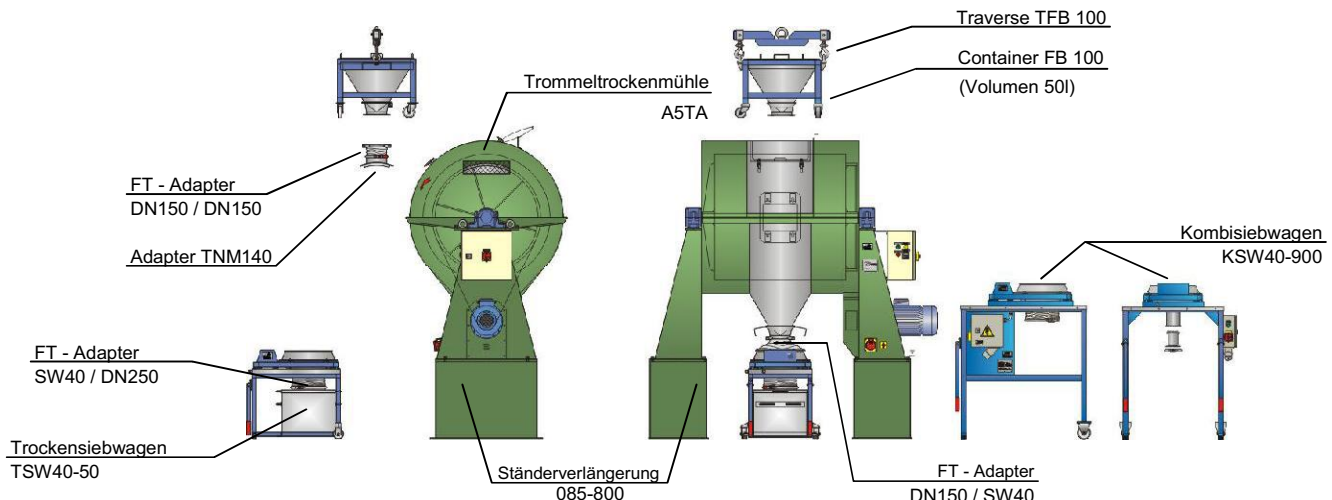
Beispiel einer Trommeltrockenmühle A5TA mit zuzuordnenden Produkten
