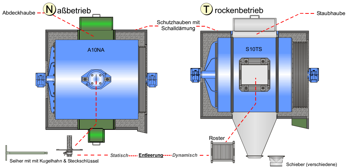
Ständerbauart
